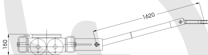
Fahrwerk (lenkbar) Nutzlast 200 kN Einzelement
