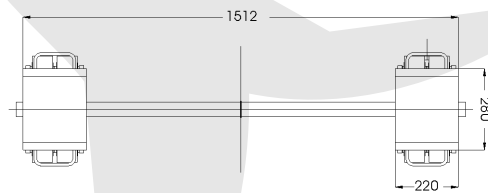
Fahrwerk (lenkbar) Nutzlast 200 kN Einzelement
