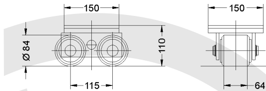
Fahrwerk (starr) Nutzlast 30 kN / Paar 15 kN / Einzelement
